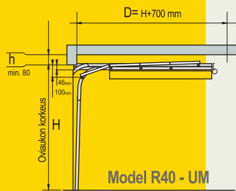
Vaatii min. 80 mm ylätilaa (h)
