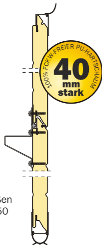
UM mit Zugfedernpaketen unterhalb montiert
