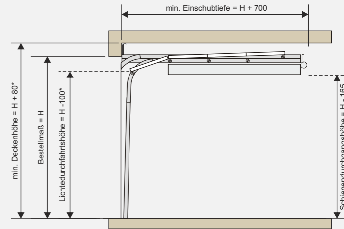
UM - Beschlagsystem mit Zugfedernpaketen unten montiert
