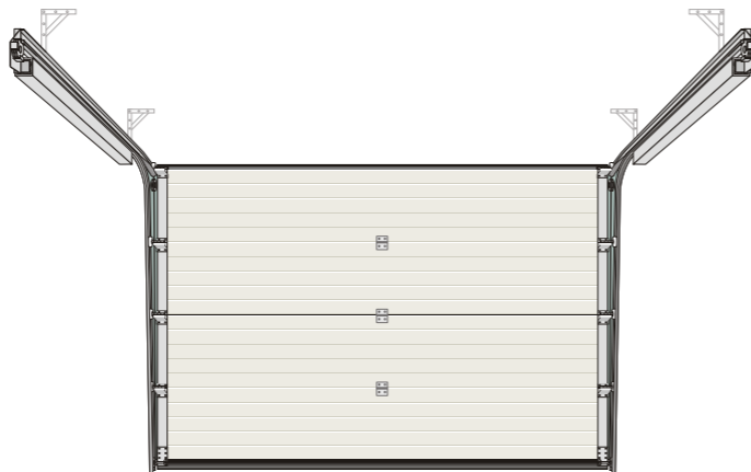
UM mit Zugfedernpaketen unterhalb montiert
