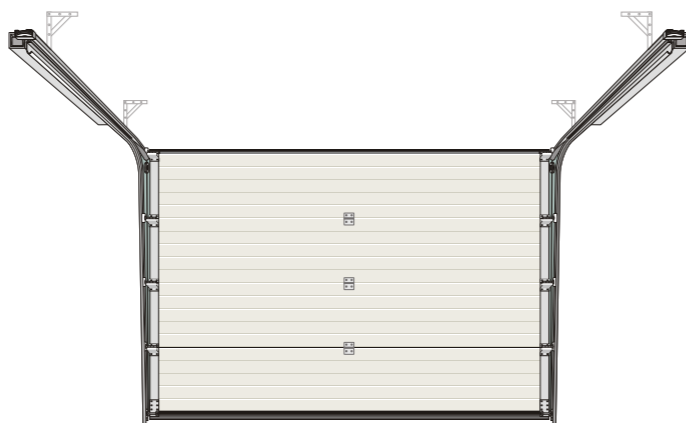
SM mit Zugfedernpaketen seitlich montiert
