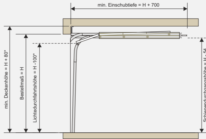
SM - Beschlagsystem mit Zugfedernpaketen seitlich montiert
